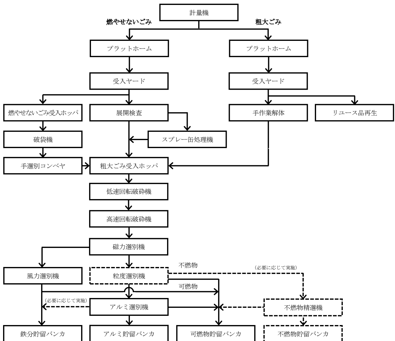
図 2.2.1 マテリアルリサイクル推進施設 基本的処理フロー（参考）
