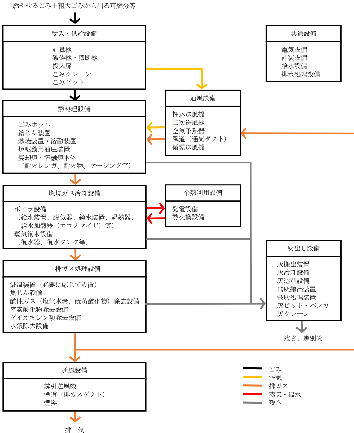
図 2.1.1 エネルギー回収型廃棄物処理施設 基本的処理フロー（参考）
