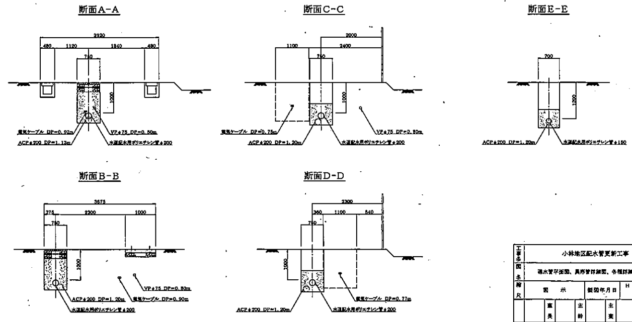
横断面図縮尺1:50
