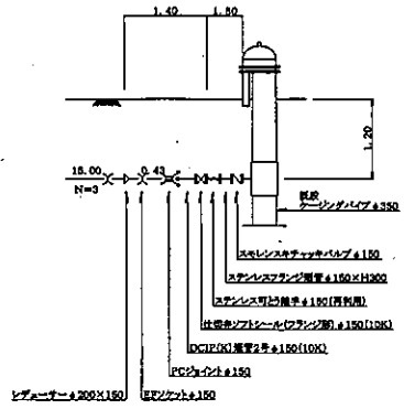
断面詳細図
