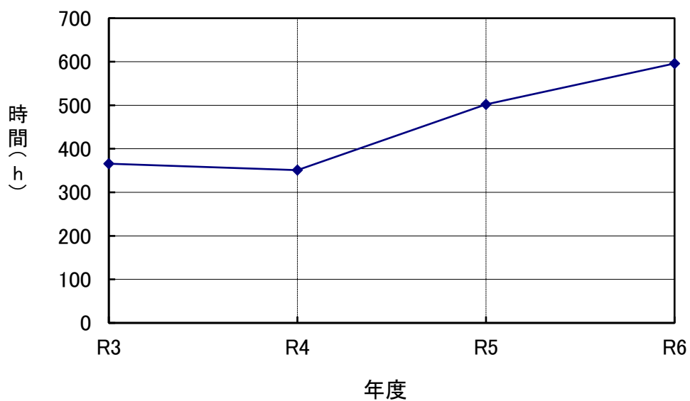
光化学オキシダント経年変化 昼間の1時間値0.06ppmの超過時間数
