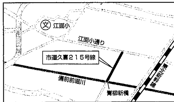
市道久喜215号線 拡幅工事箇所(北青柳)
