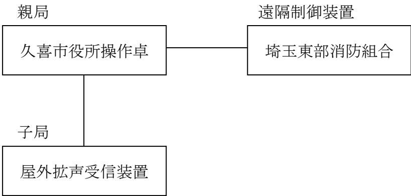
【回線構成図】
