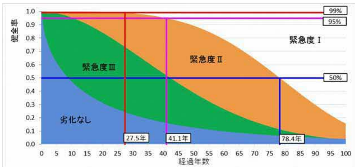
図 7-2-2 P-F 曲線による管理区分と目標基準までの年数 (劣化なし～緊急度 Ⅲ)
