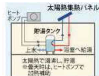
太陽熱利用給湯システム
