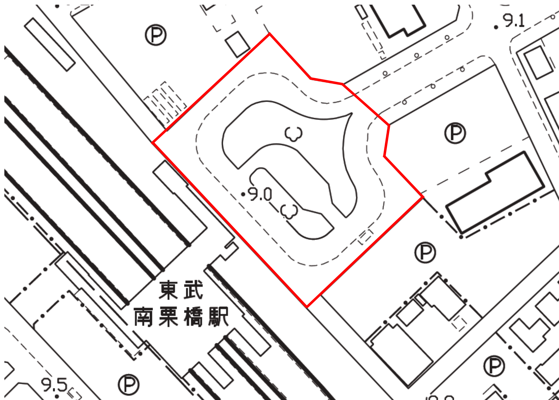
南栗橋駅東口駅前広場平面図
